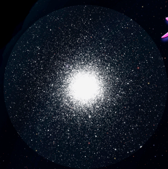
M3・球状星団 b
