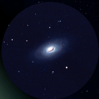
M64・黒眼銀河 a
